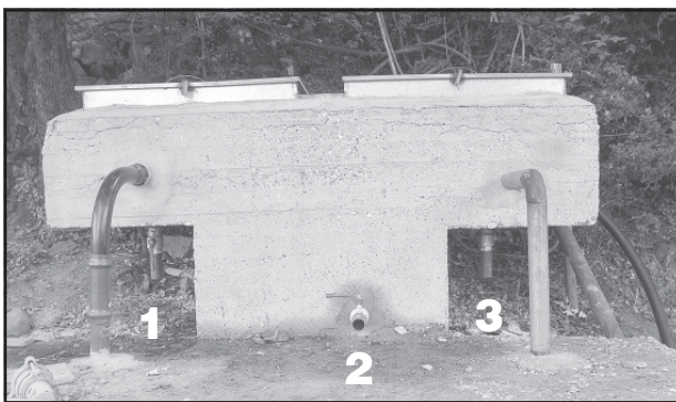
Βάνες καθαρισμού σε κάθε ένα από τα 3 φρεάτια
