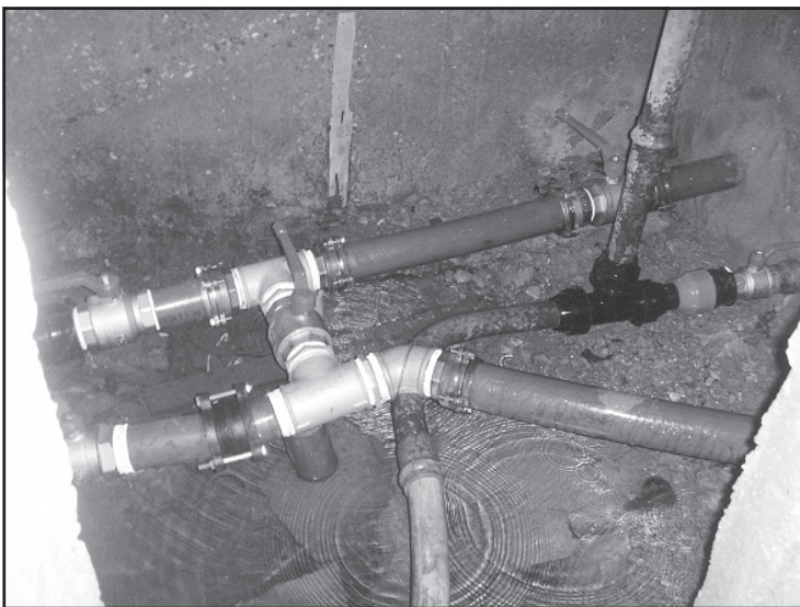
Οι καινούργιες σωληνώσεις και βάνες στις δεξαμενές.
